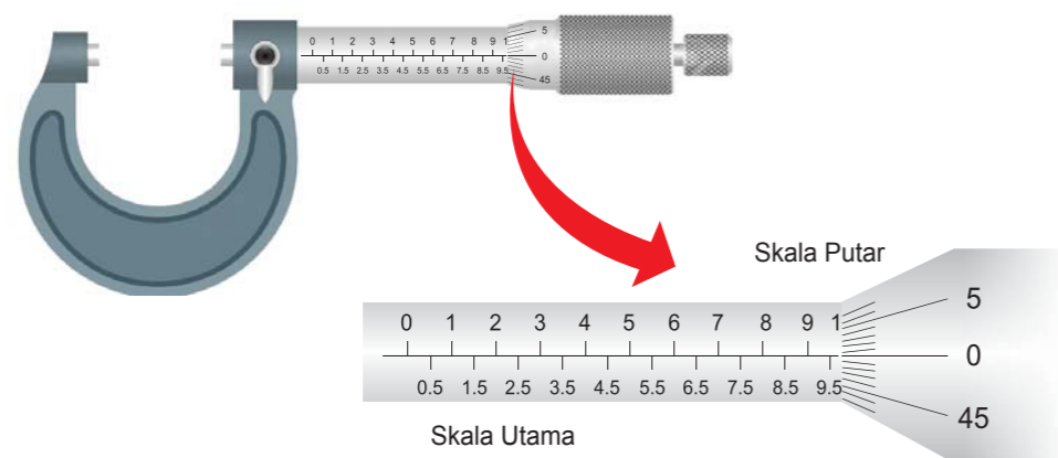
Gambar 6. Mikrometer sekrup (pada gambar menunjukkan nilai 10,00 \text{ mm} )
