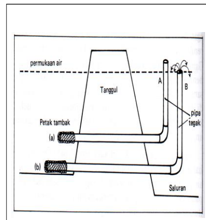
Gambar 27. Pintu pengeluaran air
