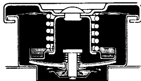
Katup vakum terbuka dan katup pelepas tertutup
