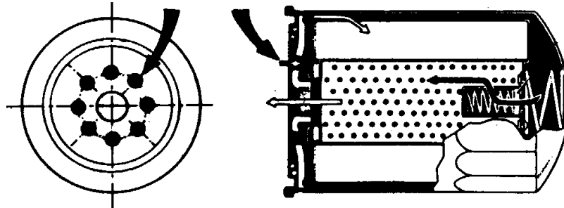
Katup anti-balik (karet)
