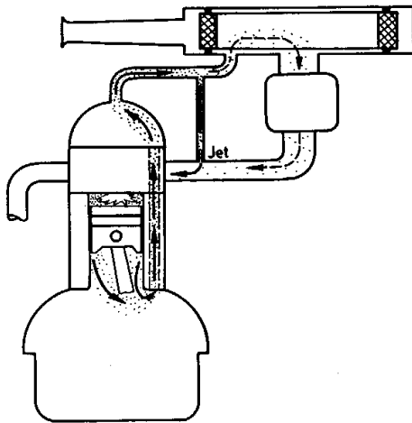
Sistem Ventilasi Sederhana
