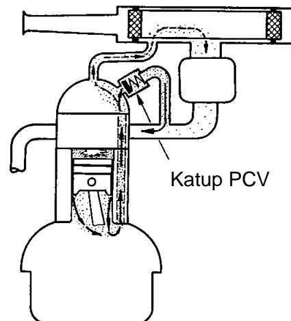
Sistem PCV
