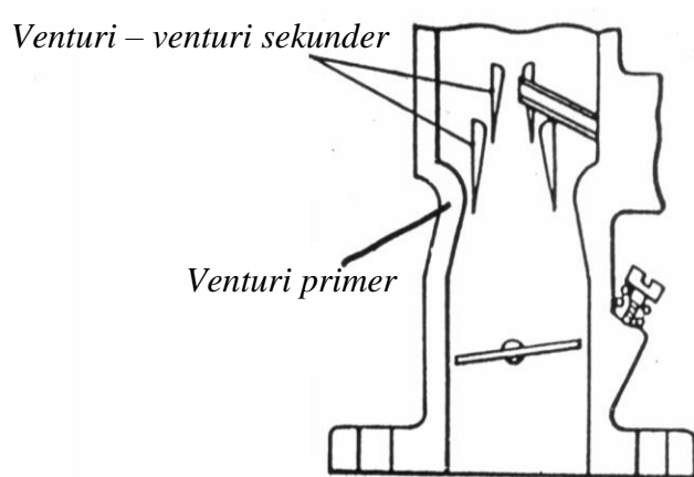
Satu venturi dengan venturi sekunder
