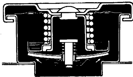
Katup pelepas terbuka dan katup vakum tertutup
