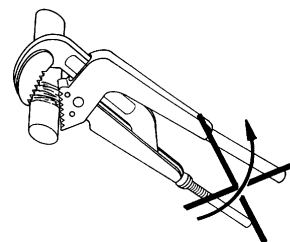
Mulut didorong : Slip Penggunaan yang SALAH
