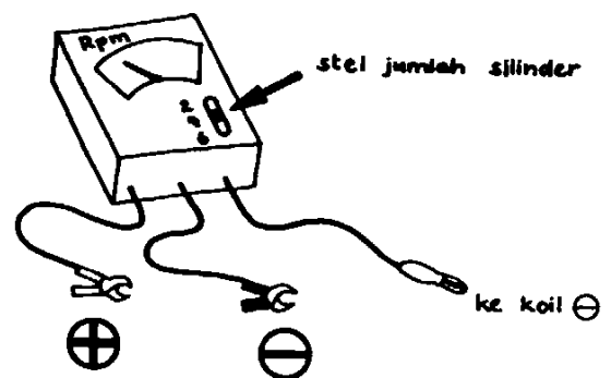
Takhometer
