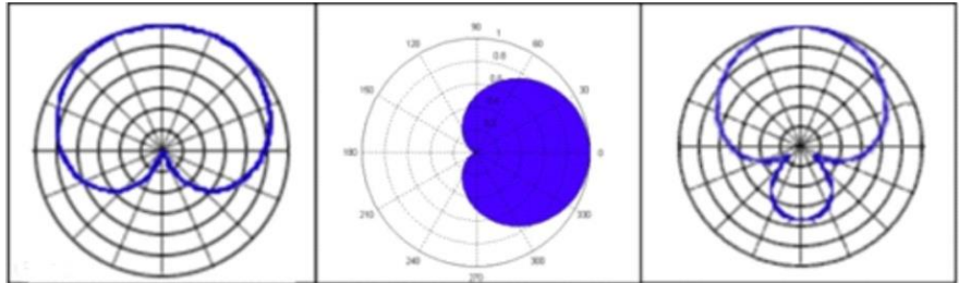
Gambar 235. Pola arah uni directional
