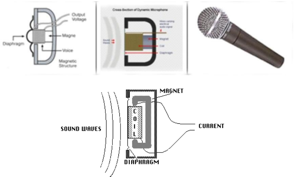
Gambar 228. Sistem kerja dynamik microphone
