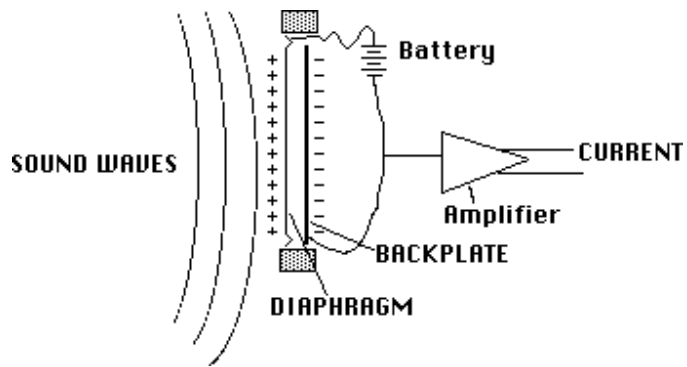
Gambar 230. Sistem kerja condensor microphone
