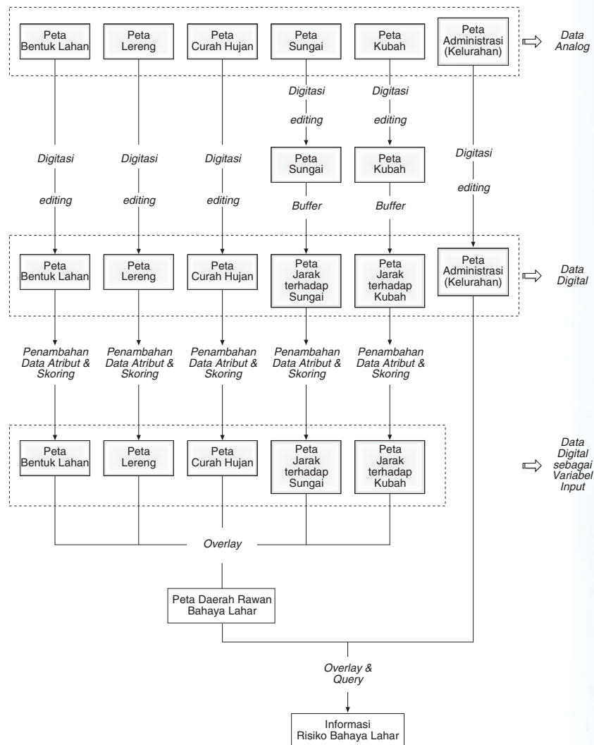
Gambar 5.9 Diagram alir model penentuan daerah rawan bahaya lahar gunung berapi.
